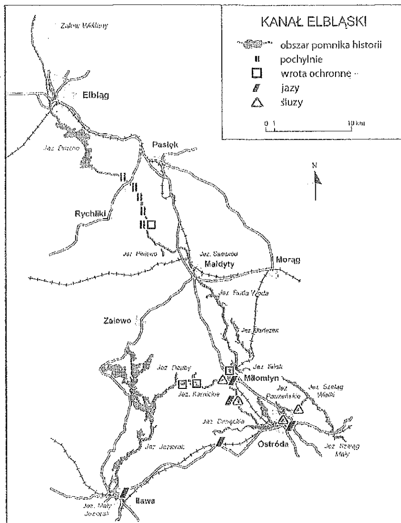
Schemat przebiegu Kanalu Elbląskiego
